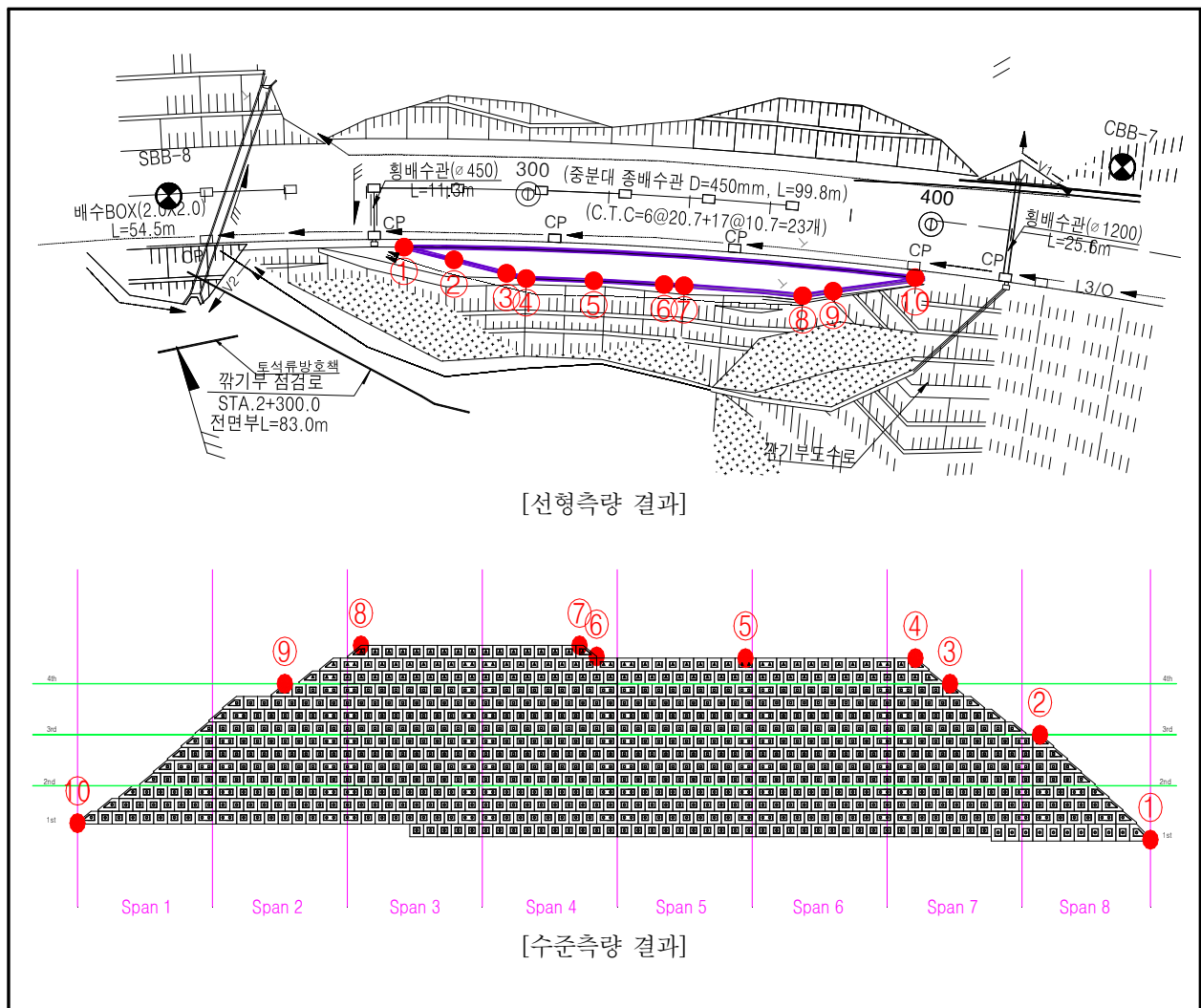
【그림 5.3.5】 선형 및 수준측량 결과
